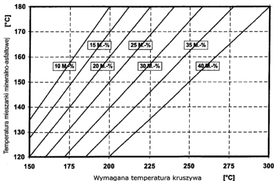
Tablica 11. Temperatura kruszywa w zależności od ilości zimnego i suchego granulaku asfaltowego
